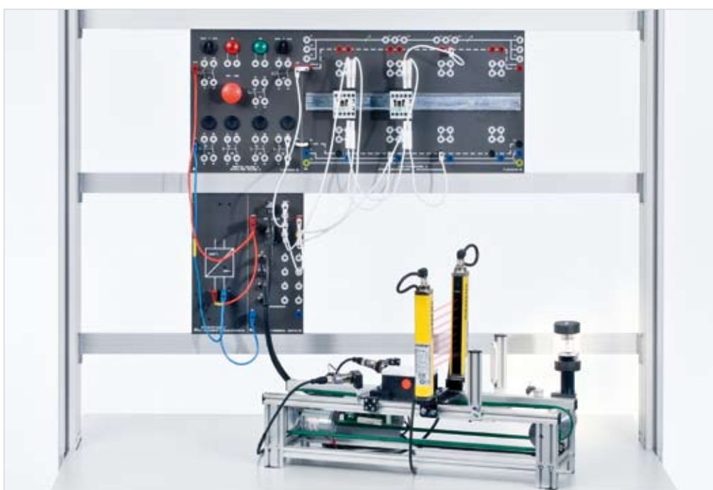
Exemple d'expérience « Systèmes de sécurité optiques CSY 4/5 »
