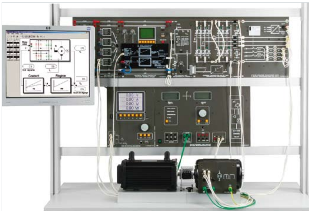
Exemple d'expérience « Régulation de la vitesse de rotation d'un moteur à courant continu EPE 11 »
