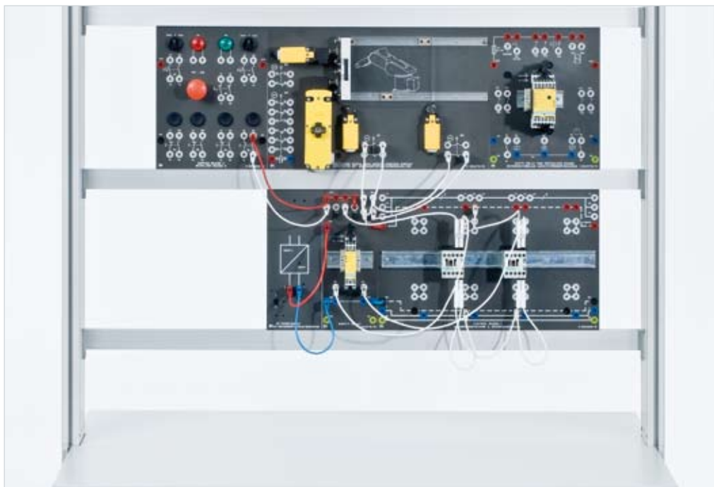
Exemple d'expérience « Circuits à relais de sécurité CSY 1 »
