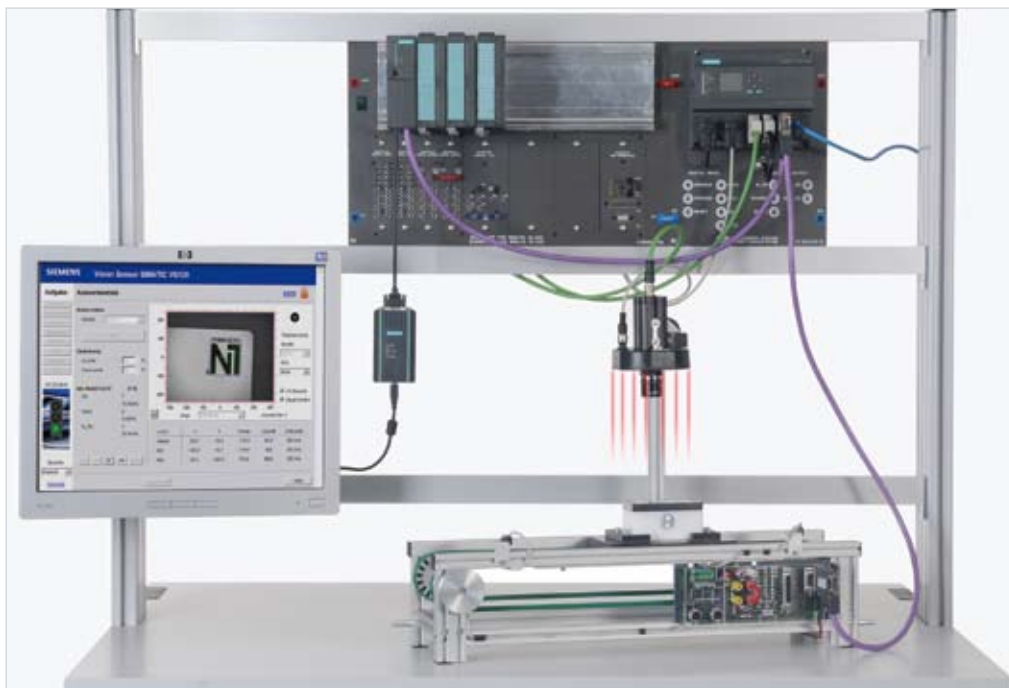
Exemple d'expérience « Traitement d'images CVS 1 »
