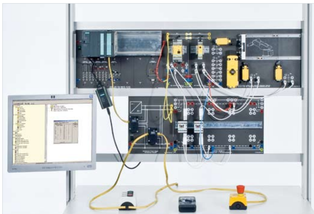
Exemple d'expérience « AS-i-Safety at work CSY 2 »
