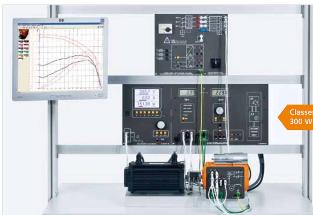
Exemple d'expérience « Moteur monophasé avec condensateurs de service et de démarrage EEM 3.4 »
