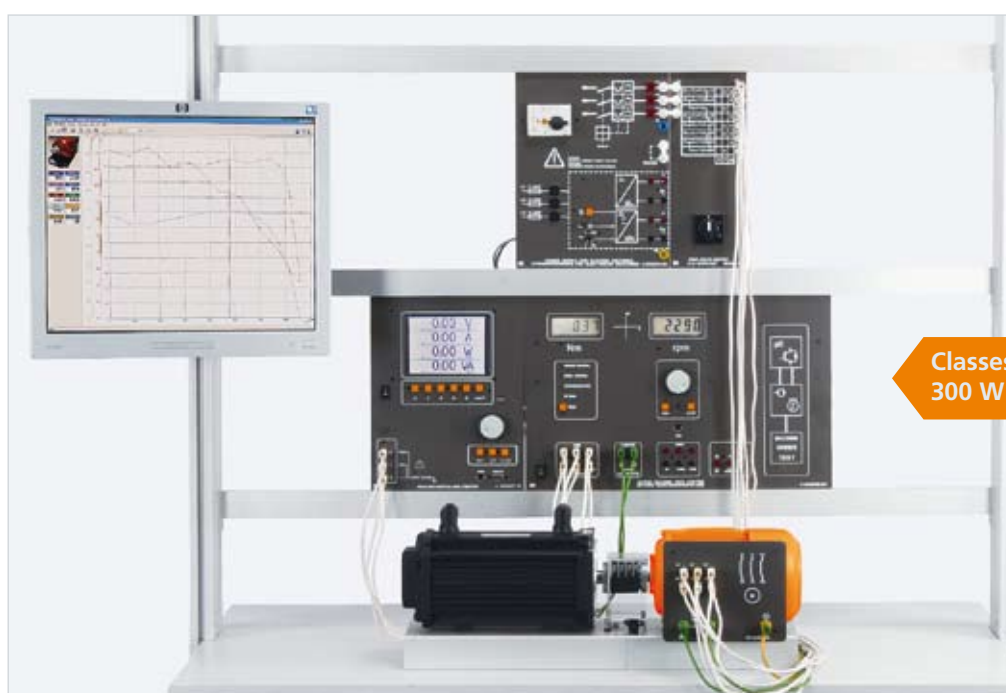
Exemple d'expérience « Moteur triphasé avec rotor à cage d'écureuil EEM 4.1 »
