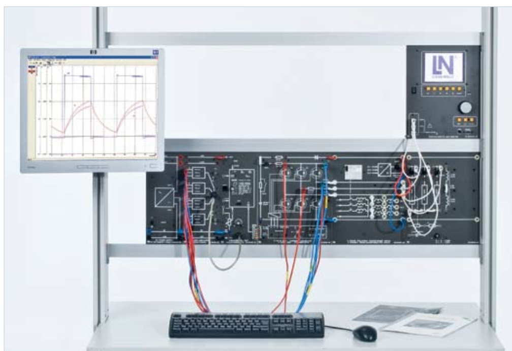
Exemple d'expérience « Convertisseurs statiques à commutation forcée EPE 20 »
