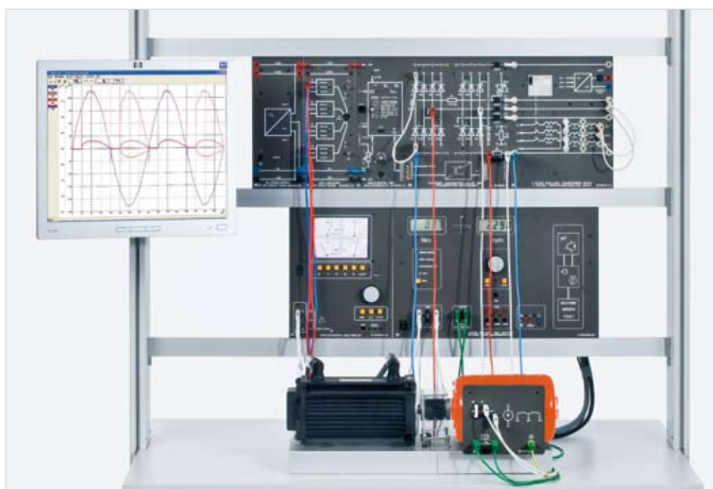
Exemple d'expérience « Entraînements par convertisseur statique avec moteurs universels EPE 16 »
