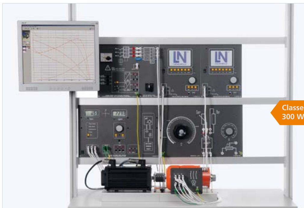
Exemple d'expérience « Moteur triphasé avec bagues collectrices EEM 4.4 »
