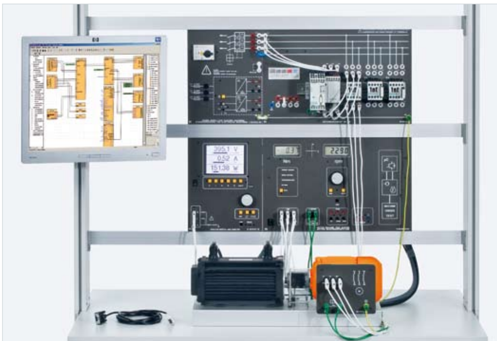
Exemple d'expérience « Relais de gestion de moteur EDT 51 »
