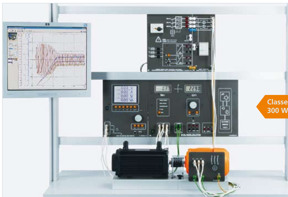
Exemple d'expérience « Démarrage en douceur avec des machines triphasées EDT 17 »
