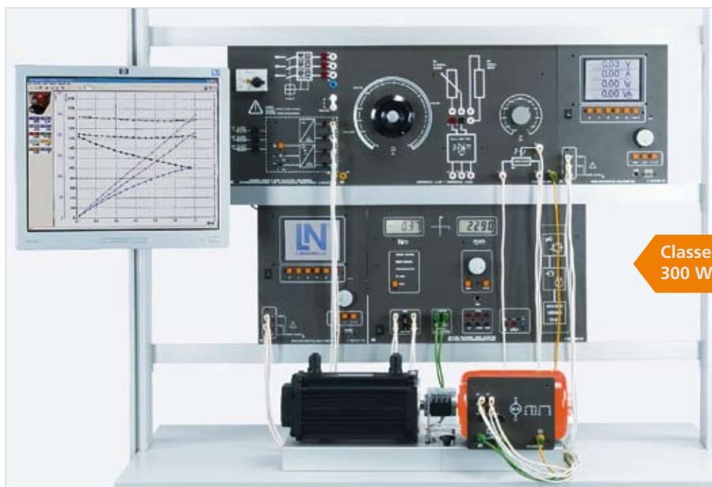
Exemple d'expérience « Machines à courant continu EEM2 »
