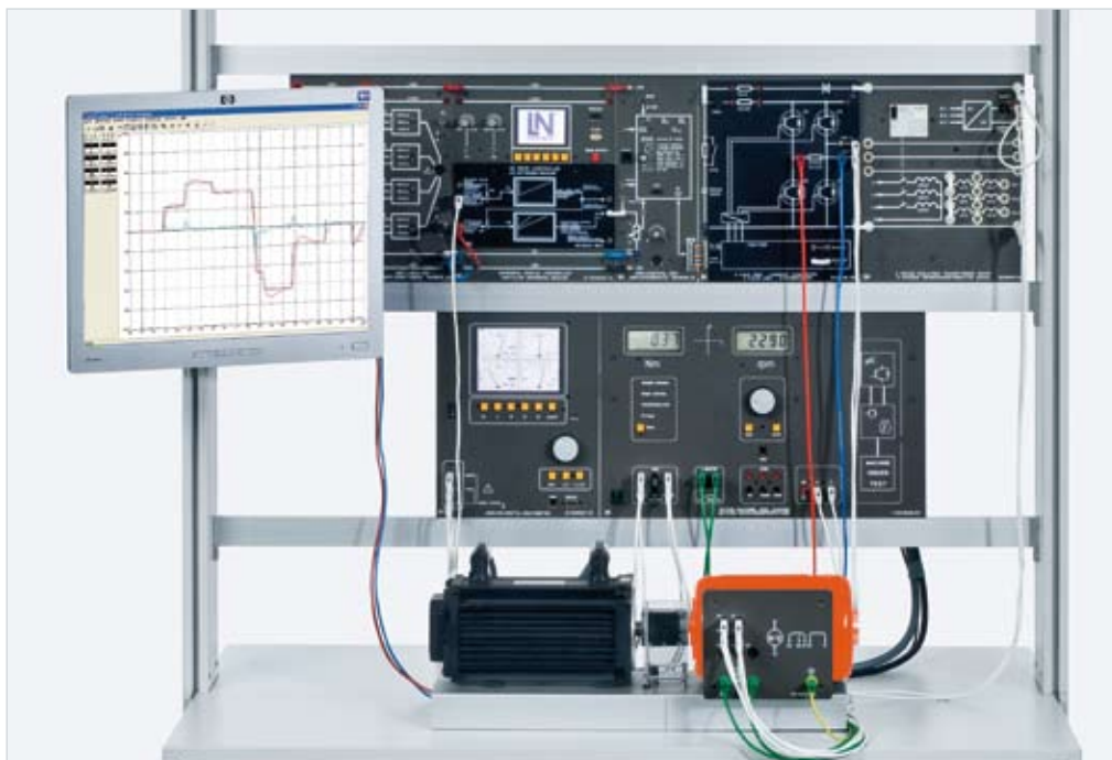
Exemple d'expérience « Entraînements à courant continu avec modulation de largeur d'impulsions EPE 21 »
