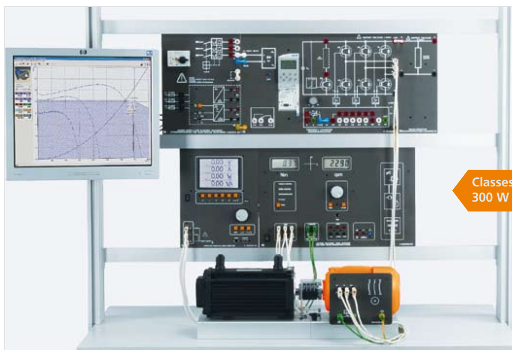
Exemple d'expérience « Commandes avec convertisseur de fréquence EDT 25 »
