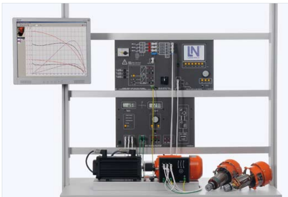
Jeu de machines triphasées décomposable EEM 10
