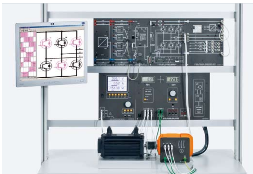
Exemple d'expérience « Convertisseurs de fréquence avec moteur asynchrone triphasé EPE 26 »
