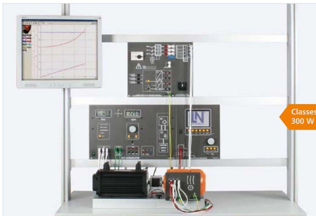
« Machine à réluctance triphasée EEM 5.3 »
