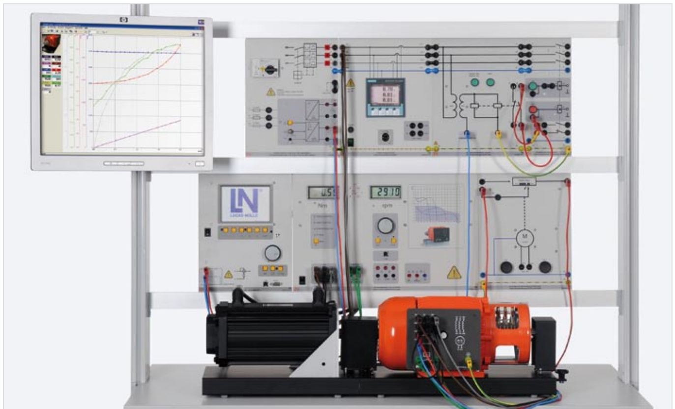
Versuchsbeispiel „Generatorschutz- Läufererdschlussschutz EGP 3“
