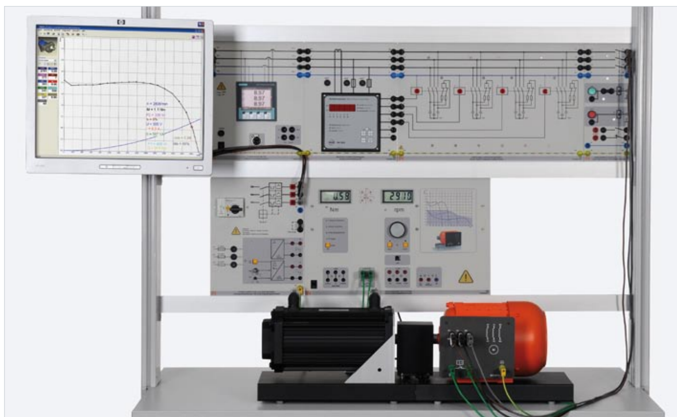
Versuchsbeispiel „automatische Blindleistungskompensation EUC 3“
