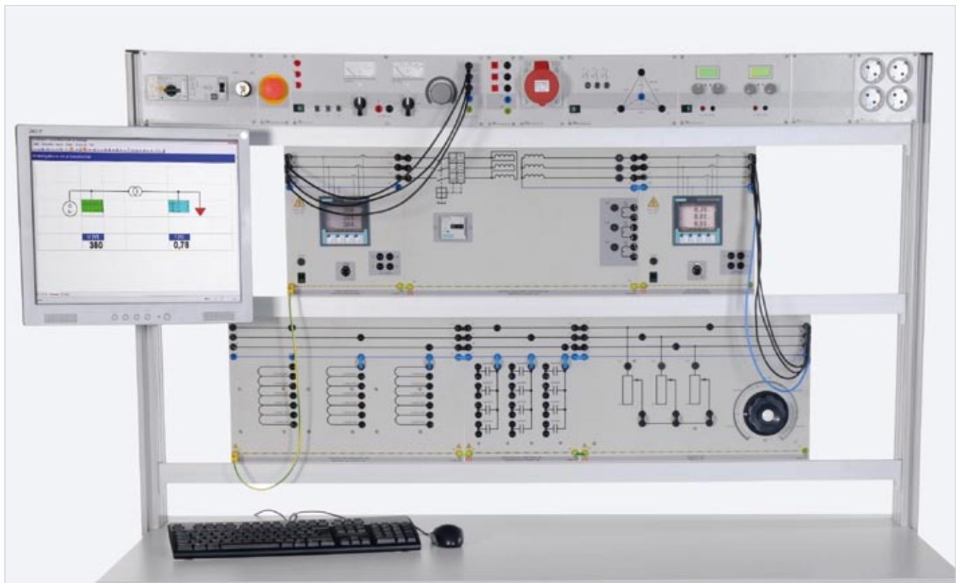
Versuchsbeispiel „Untersuchungen an Transformatoren EUT“
