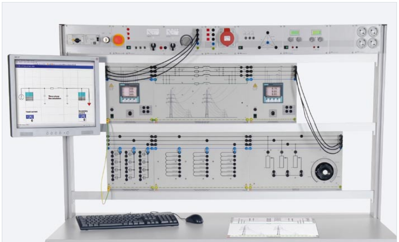
Versuchsbeispiel „Untersuchungen an Drehstromleitungen EUL 1“
