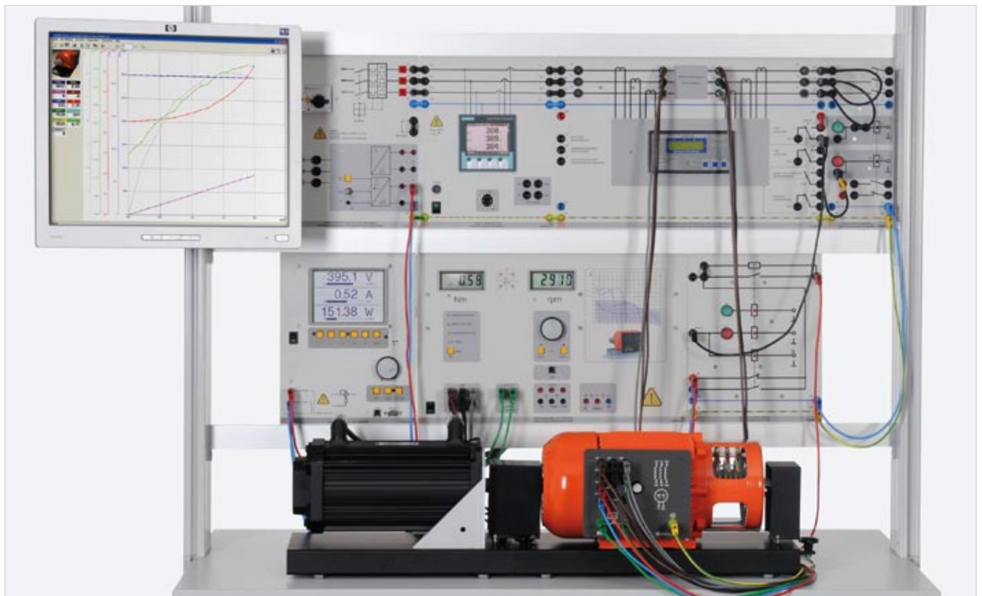
Versuchsbeispiel „Generator-Differentialschutz EGP 2“
