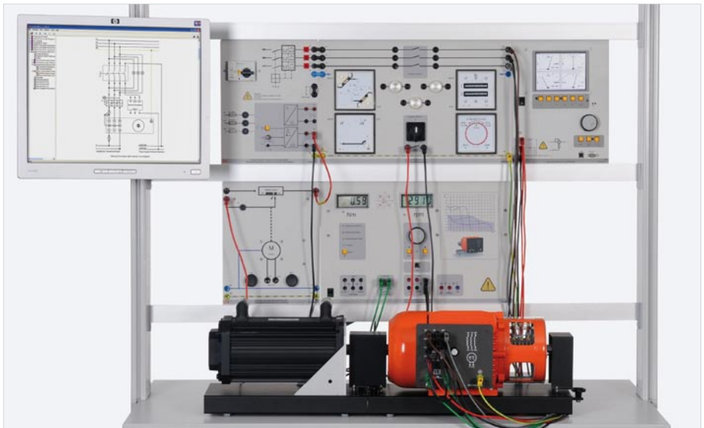
Versuchsbeispiel „Handbetätigte Synchronisierschaltungen EUG 1“
