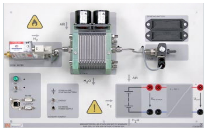
50-VA-Brennstoffzellen-Stack
