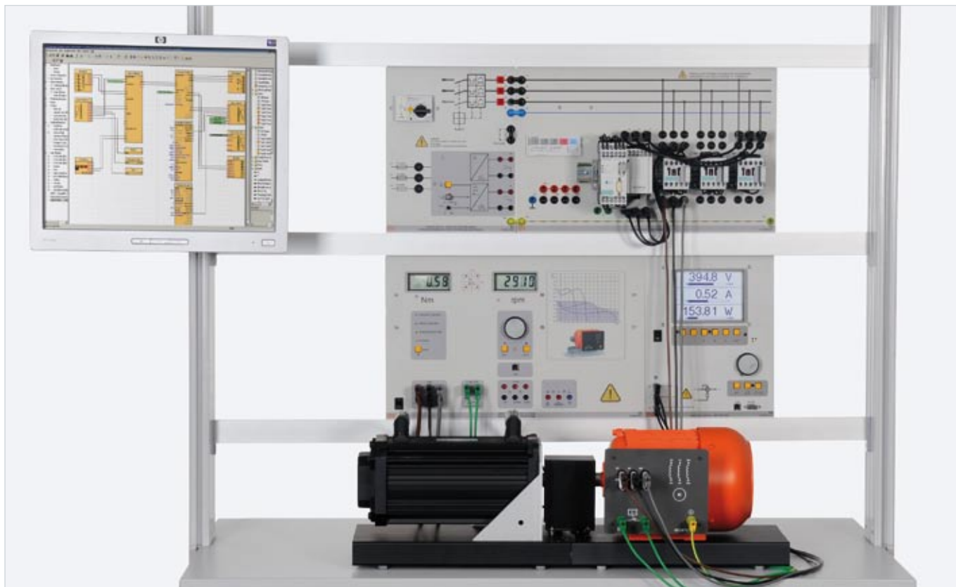
Versuchsbeispiel „Motormanagementrelais EDT 51“
