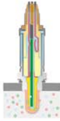
Zirkondioxidsonde
